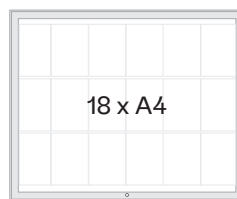
VI.CL.18.V (šxv) 1330x1080 mm
